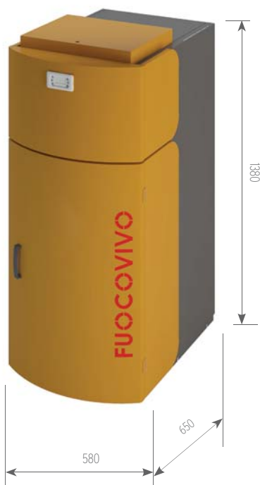
Imagen y dimensiones del modelo Compact 19KW
